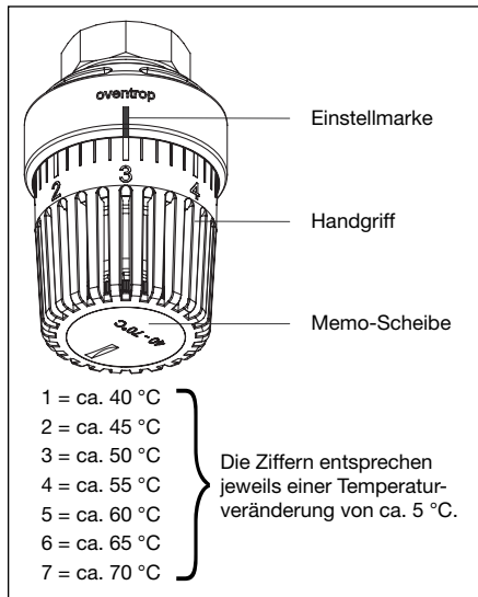
Abb. 8.3 Einstellung Trinkwassertemperatur
