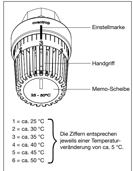
Abb. 8.4 Einstellung Vorlauftemperatur Heizkreis
