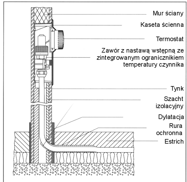
"Unibox E plus", głębokość zabudowy 57 mm
