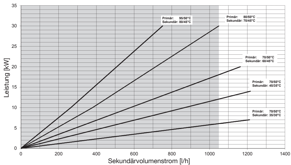
Abb. 7: Leistungsdigramm; empfohlener max. Volumenstrom Regudis H in Verbindung mit Regumat S
