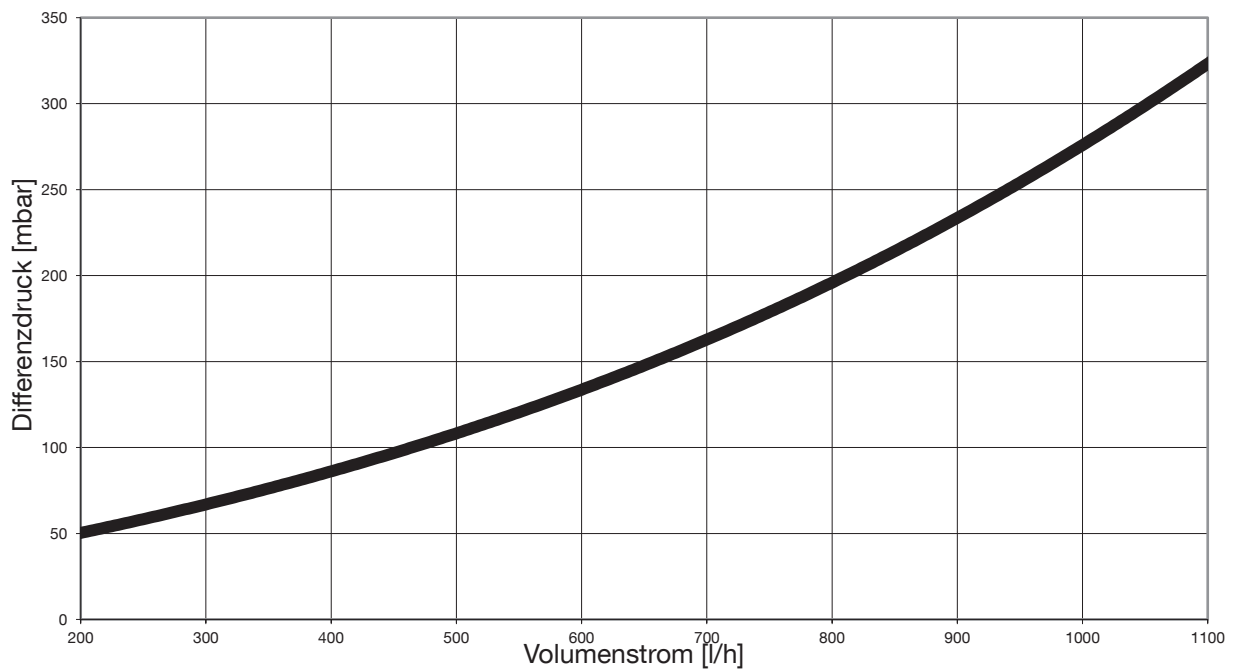
Abb. 5: Druckverlust Sekundärkreis Regudis H
