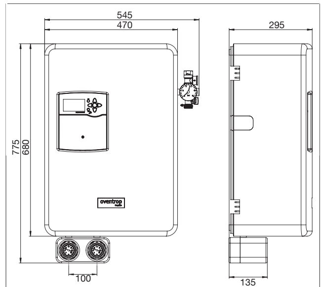
Abb. 3: Abmessungen in mm
