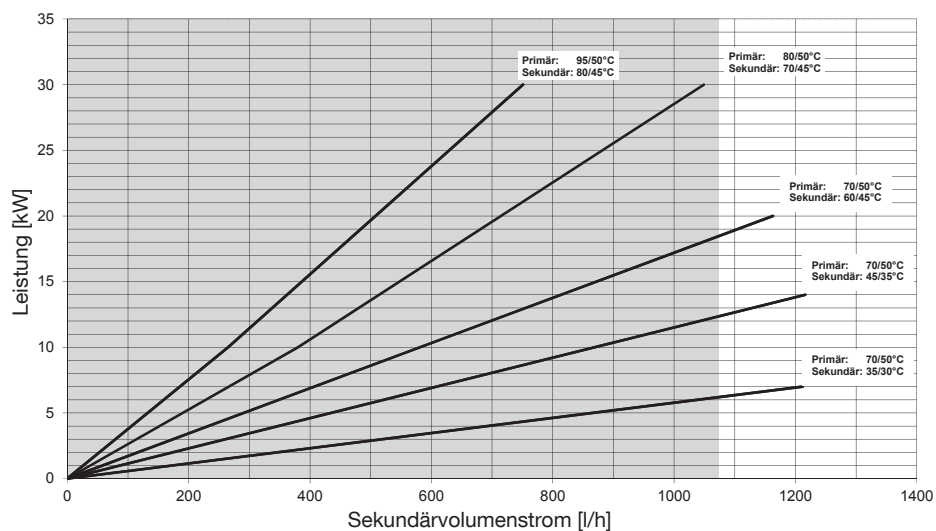
Abb. 8: Leistungsdigramm; empfohlener max. Volumenstrom Regudis H in Verbindung mit Regumat M
