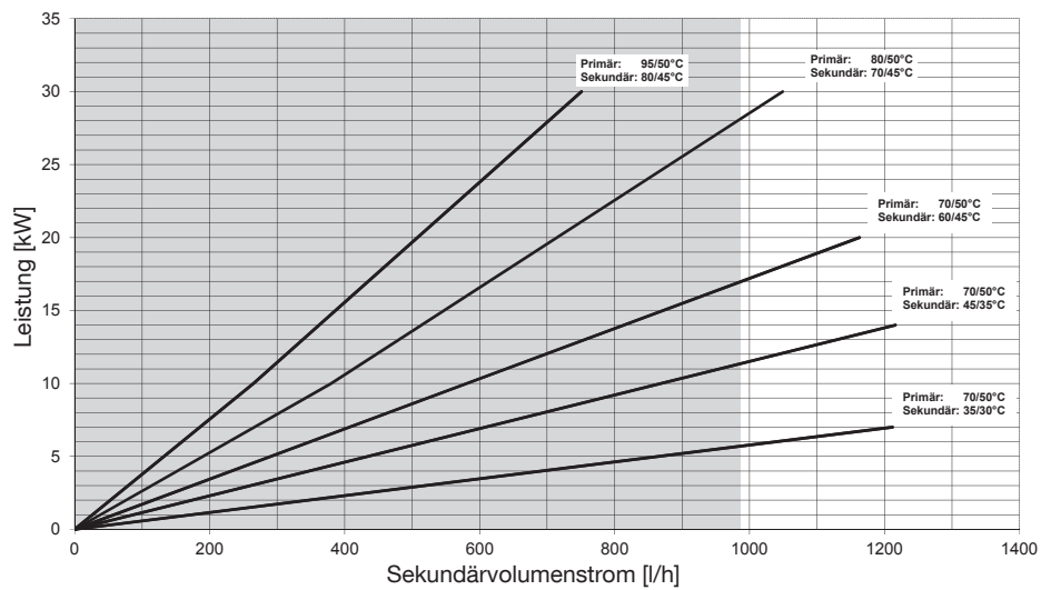
Abb. 6: Leistungsdigramm; empfohlener max. Volumenstrom Regudis H in Verbindung mit Umschaltmodul
