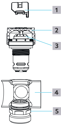
Fig. 3: Construction du mécanisme QM
