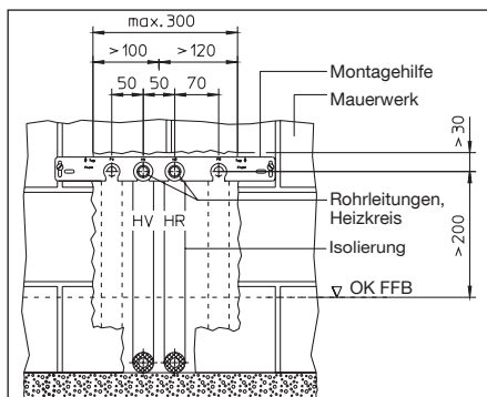
Abb. 8 Wandansicht, Heizkreisanschluss
