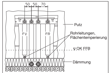
Abb. 10 Wandansicht, Flächentemperierung
