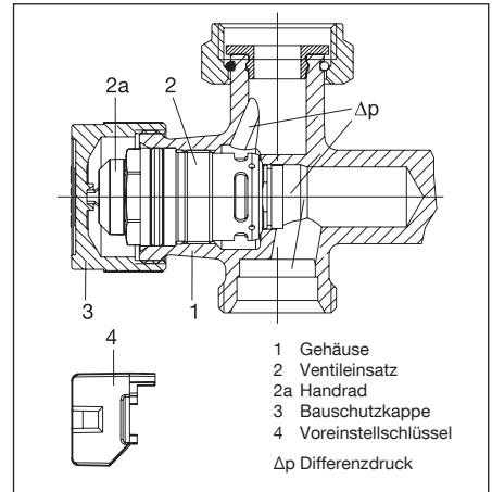
Abb. 5 Aufbau Thermostatventil (Prinzipdarstellung)
