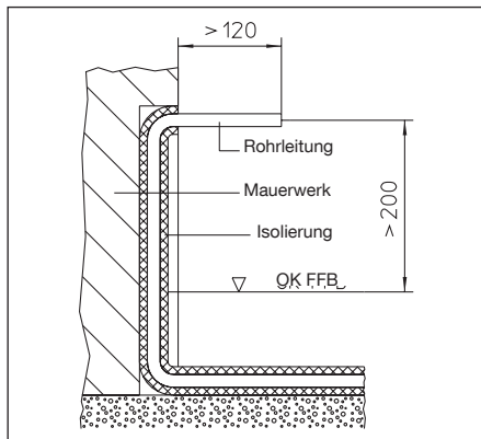
Abb. 7 Schnitt, Heizkreisanschluss
