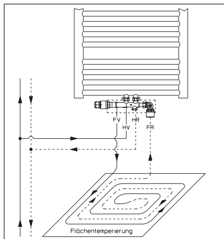
Abb. 6 Anschlusschema
