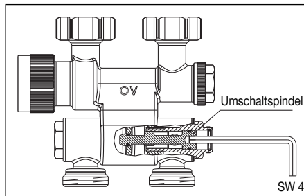
Abb. 5 Umschalten auf Einrohrbetrieb
