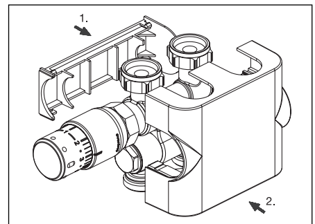
Abb. 8 Montage Design-Abdeckung
