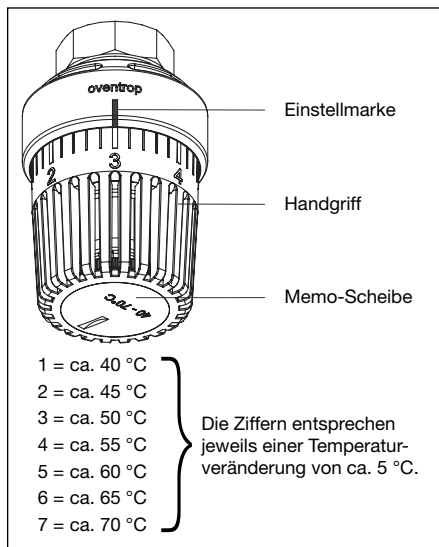
Abb. 8.3 Einstellung Trinkwassertemperatur
