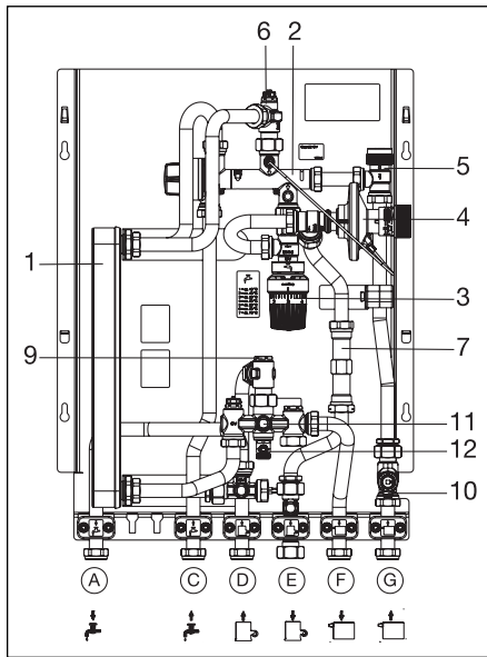
Abb. 5.1 Aufbau
