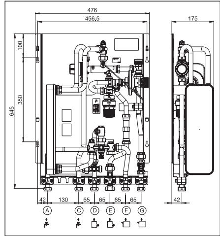
Fig. 4.1 Encombrements
