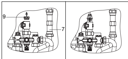
Fig. 6.2 Montage de la sonde pour compteur de calories
