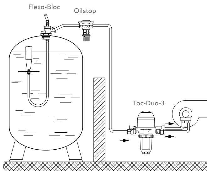
Schéma d'installation
