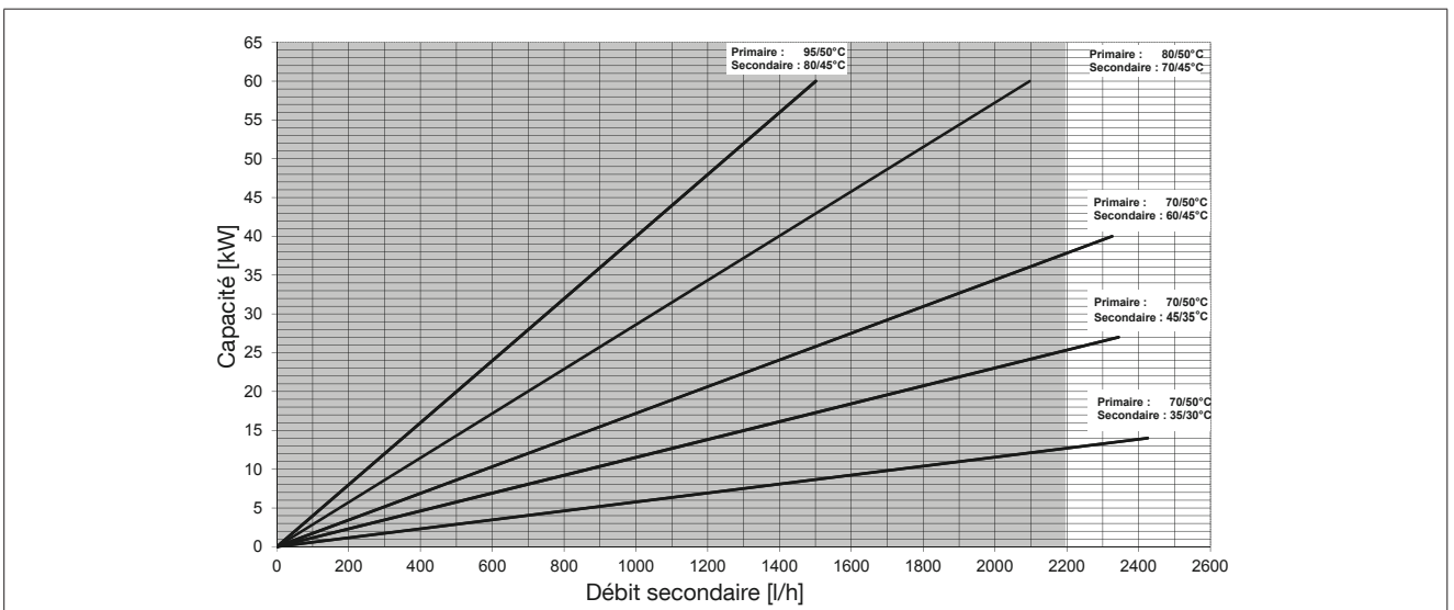
Fig. 8: Diagramme des puissances ; débit max. recommandé Regudis H en combinaison avec Regumat M3
