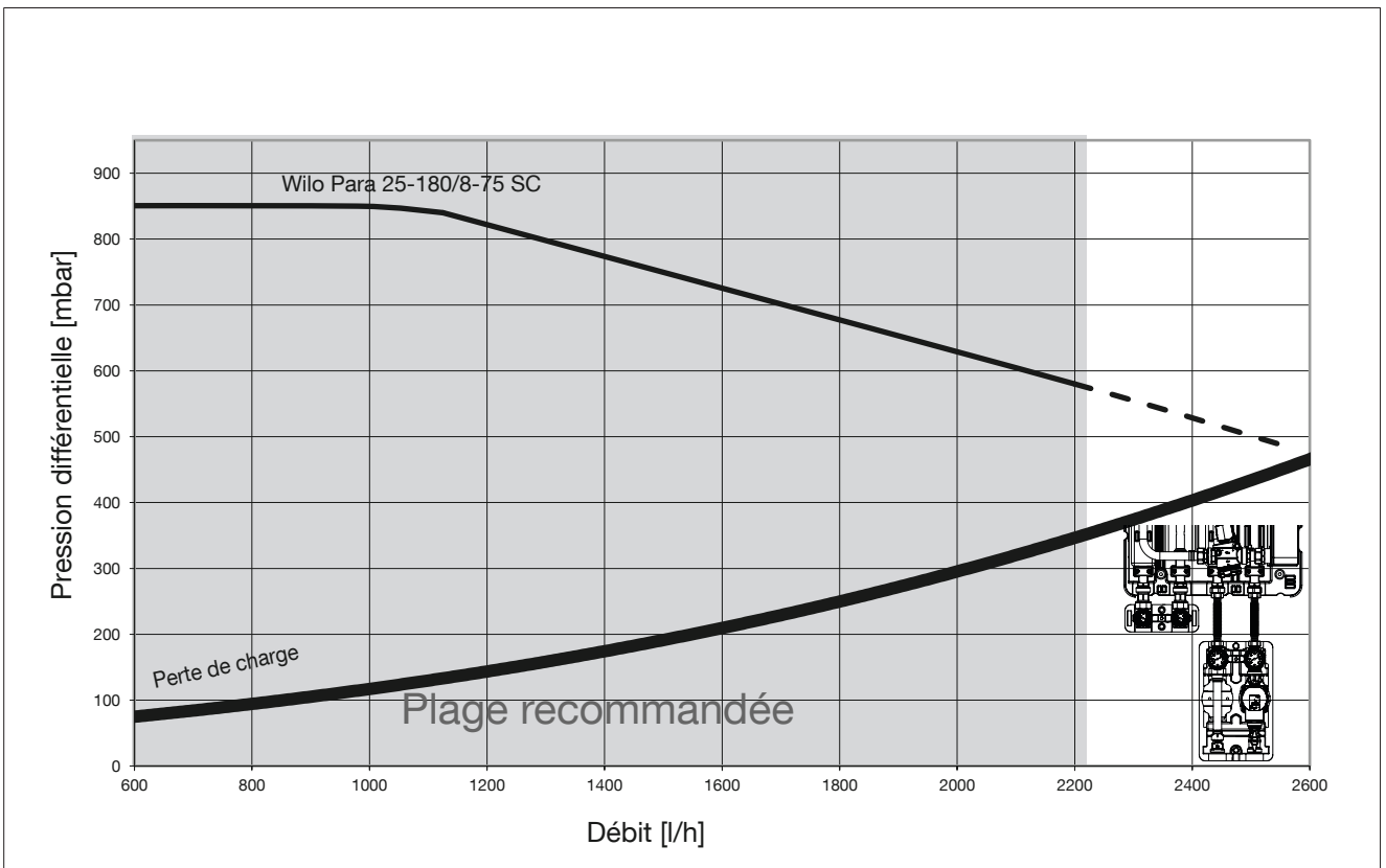
Fig. 5: Perte de charge circuit secondaire Regudis H-H
