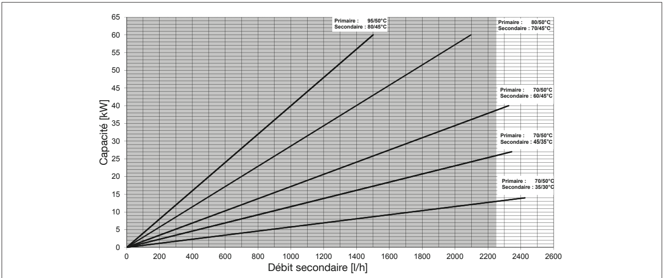
Fig. 7: Diagramme des puissances ; débit max. recommandé Regudis H en combinaison avec Regumat S
