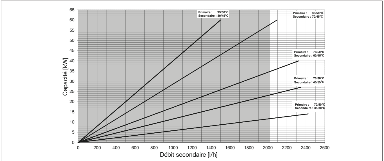
Fig. 6: Diagramme des puissances ; débit max. recommandé Regudis H en combinaison avec le module de commutation HT
