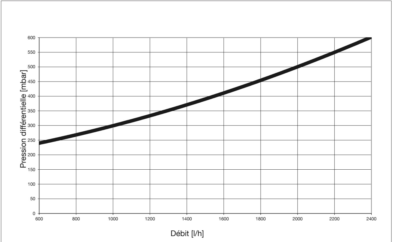
Fig. 4: Perte de charge circuit primaire Regudis H
