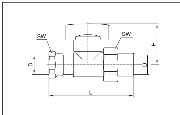
Réf. 301 19 04-08 (DN 15 à DN 25, brut)
