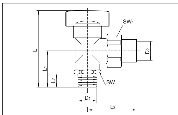
Réf. 301 49 52-54 (DN 15 à DN 25)
