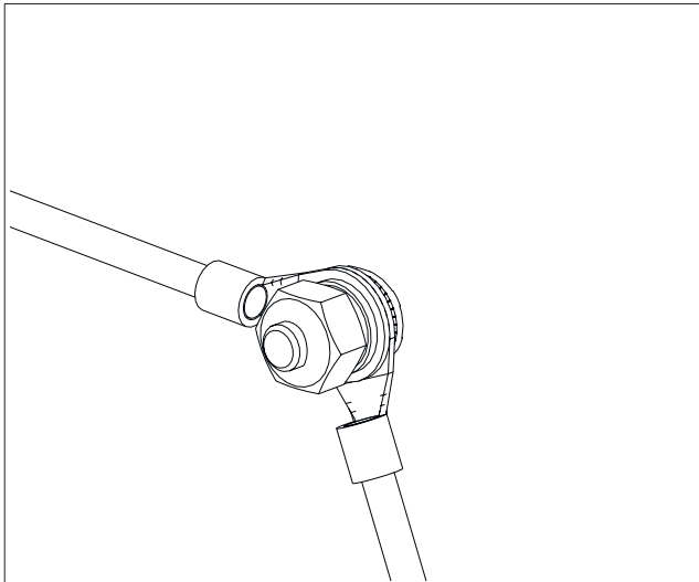
Abb. 10: Zentraler Erdungspunkt mit Verbindung zur Potentialausgleichsschiene des Gebäudes und zur Tür des Aufputzschrankes
