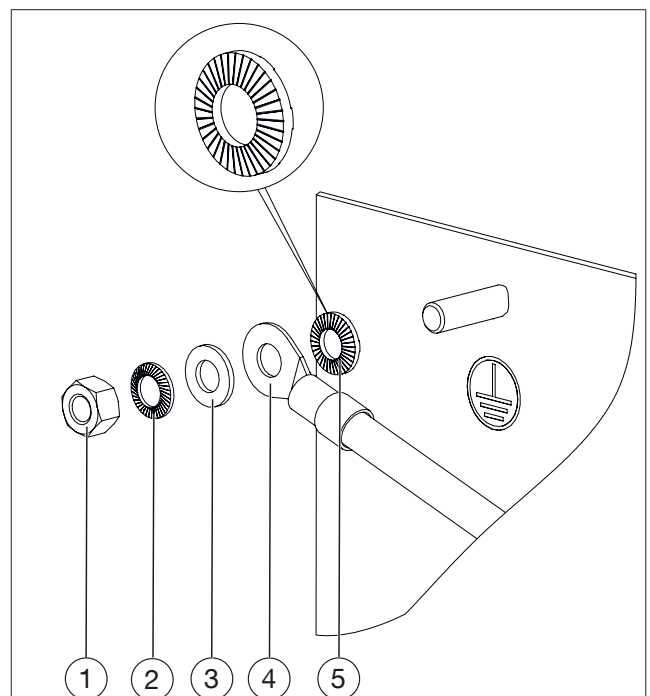
Abb. 9: Aufbau des Erdungspunktes
