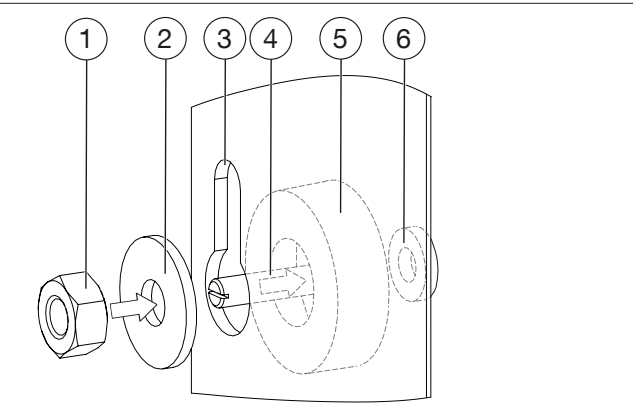
Fig. 5: Points de fixation de la station d'appartement Regudis W-HTU
