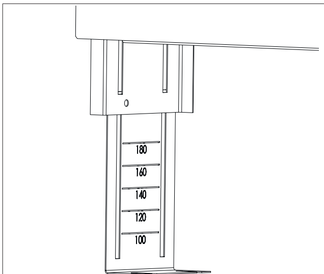
Abb. 4: Höhenmarkierung
