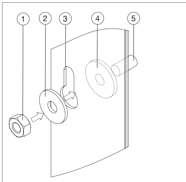
Abb. 6: Montage Befestigungspunkte „Regudis W-HTF“
