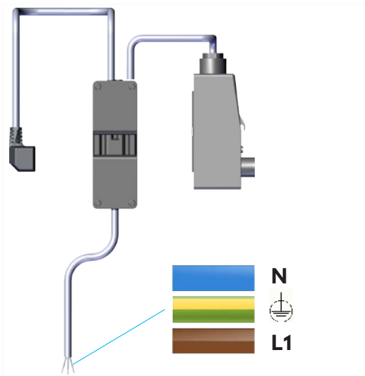
Abb. 7: Adernbelegung
