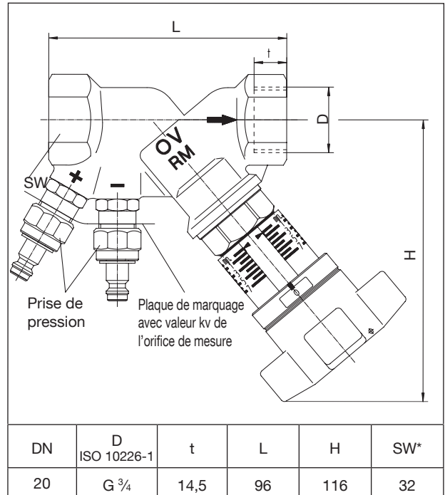
« Hydrocontrol STR » avec filetage femelle selon EN 10226 des deux côtés
