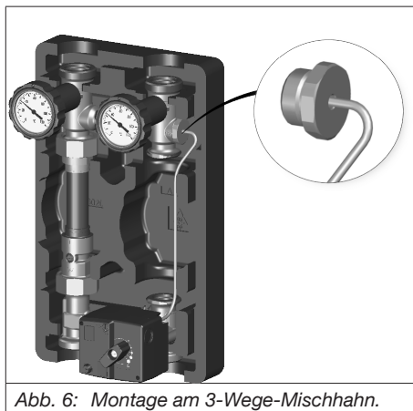
Abb. 6: Montage am 3-Wege-Mischhahn.
