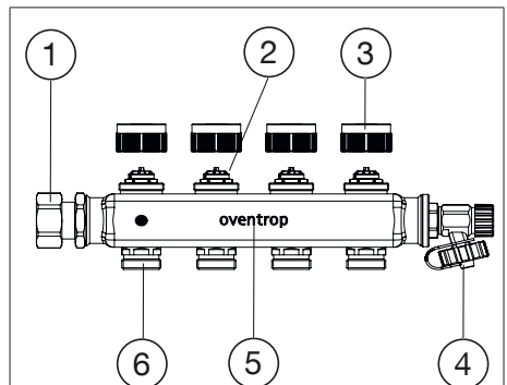
Abb. 2: Aufbau Rücklauf
