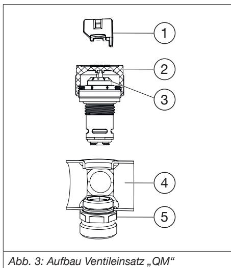
Abb. 3: Aufbau Ventileinsatz „QM“
