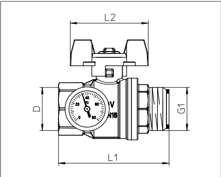
Abb. 8: Maße Kugelhahn
