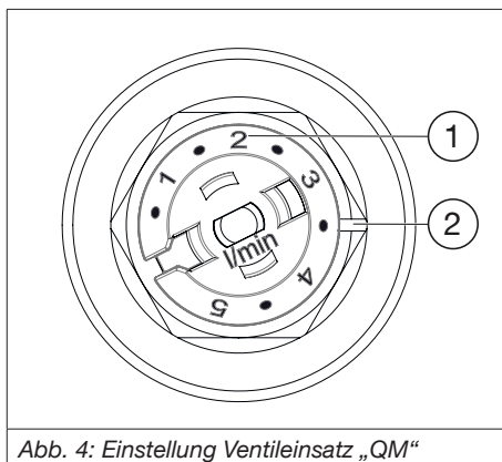
Abb. 4: Einstellung Ventileinsatz „QM“
