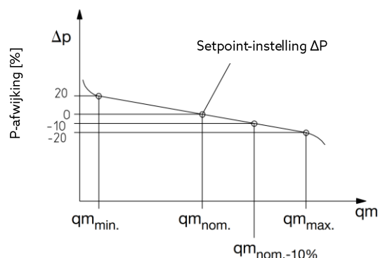
Kleinste drukafwijking bij gemiddelde instelwaarde ( q_{m\text{nom}} )
