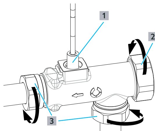
Fig. 26: Montage du capteur de débit
