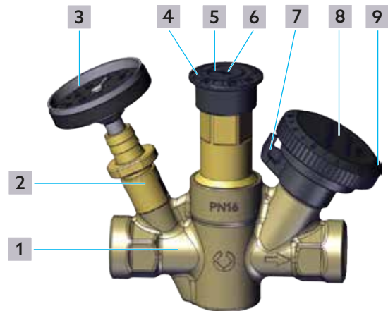
图 1： 结构
