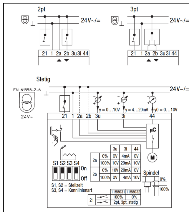
Schaltpläne, Art.-Nr. 1158031/32
