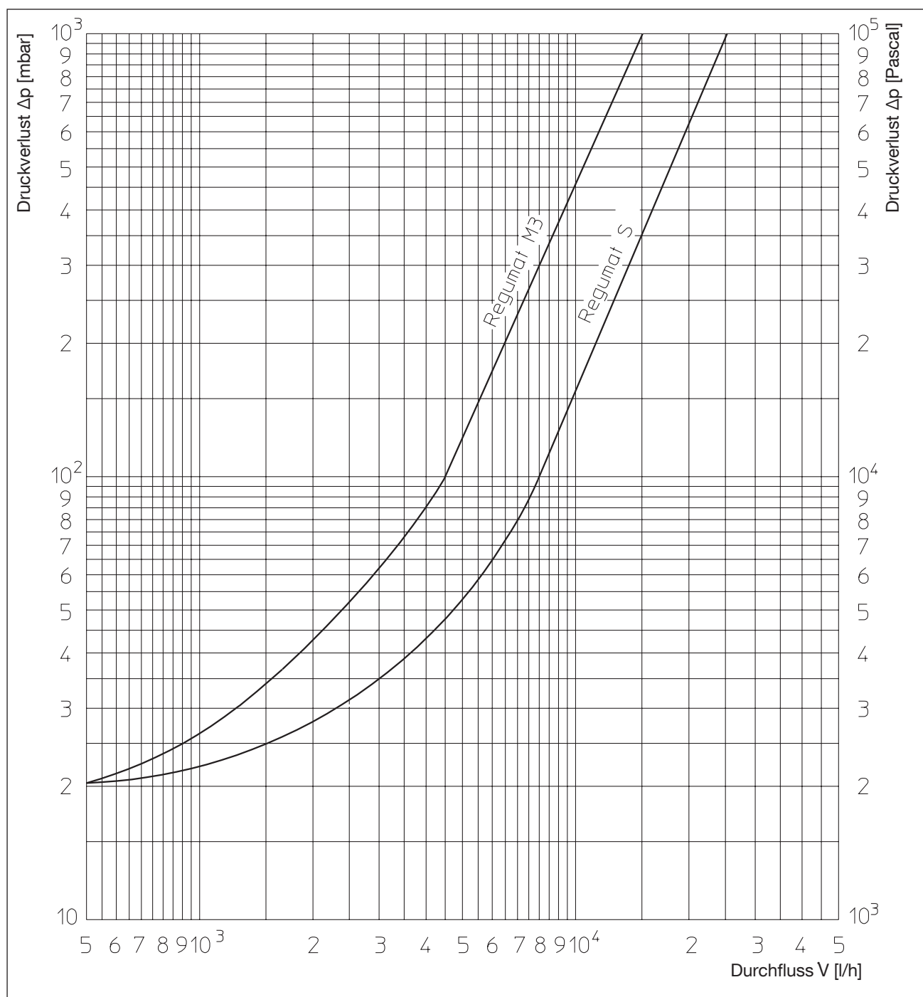
Durchflussdiagramm
