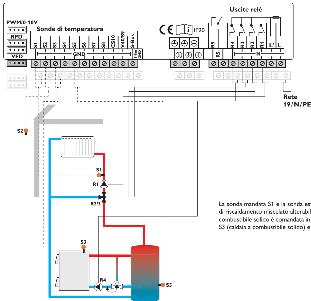
Schema 8: un circuito di riscaldamento miscelato con caldaia a combustione solido
