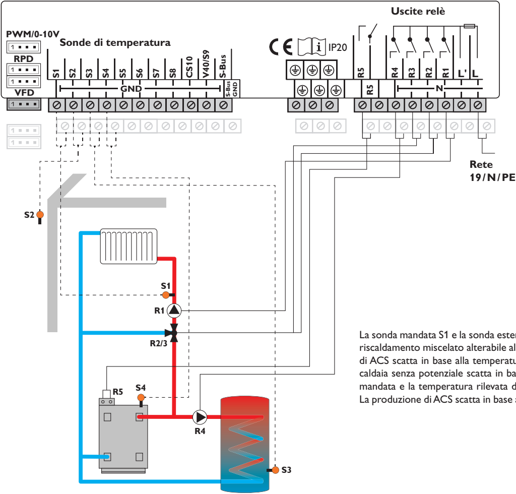
Schema 5: un circuito di riscaldamento miscelato con produzione di ACS e riscaldamento integrativo (richiesta per il circuito di riscaldamento e l'ACS)
