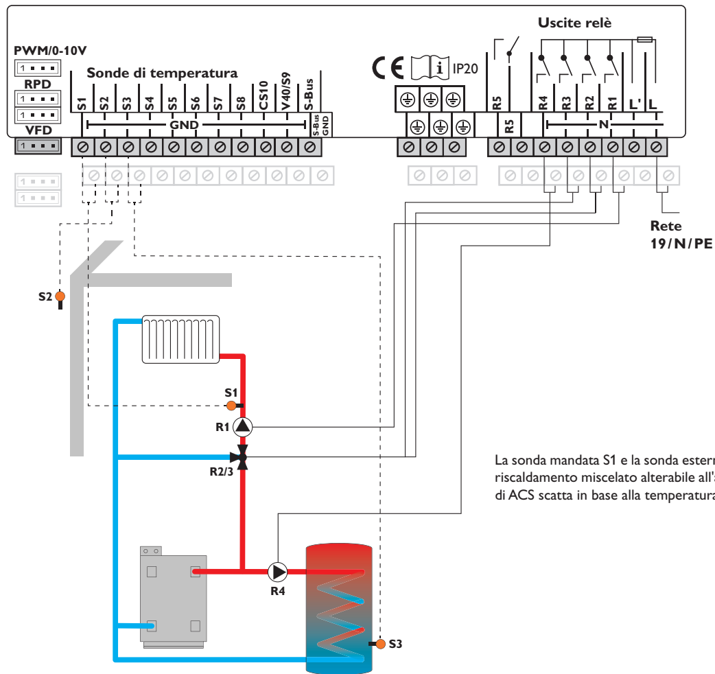
Schema 4: un circuito di riscaldamento miscelato con produzione di ACS
