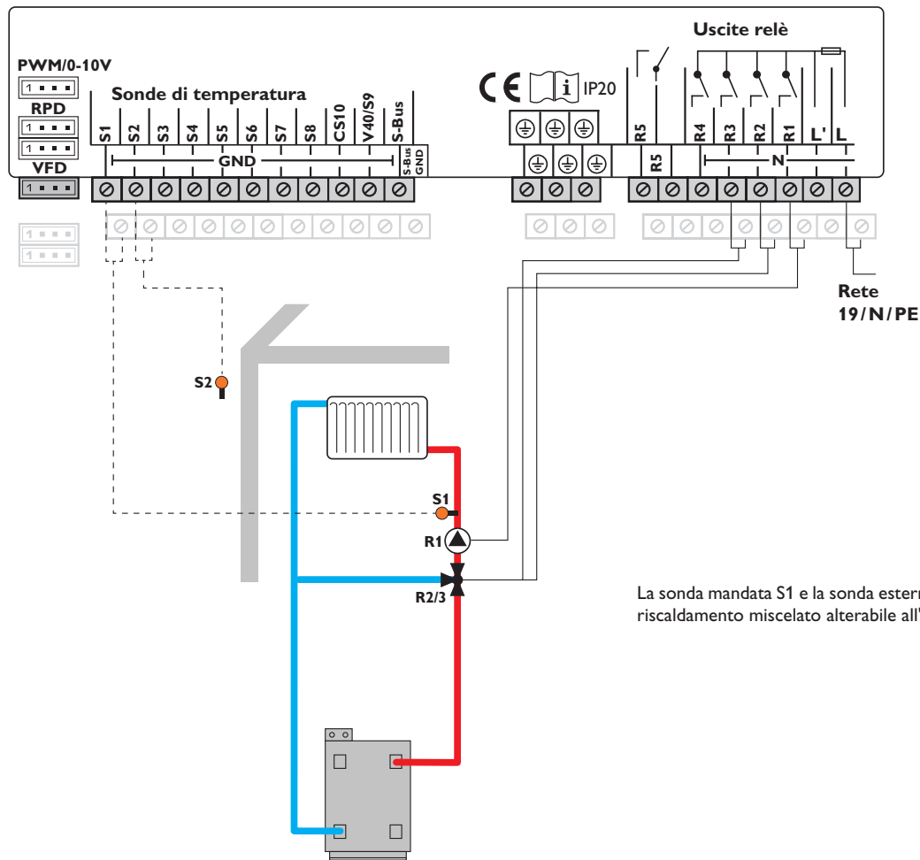
Schema 1: un circuito di riscaldamento miscelato
