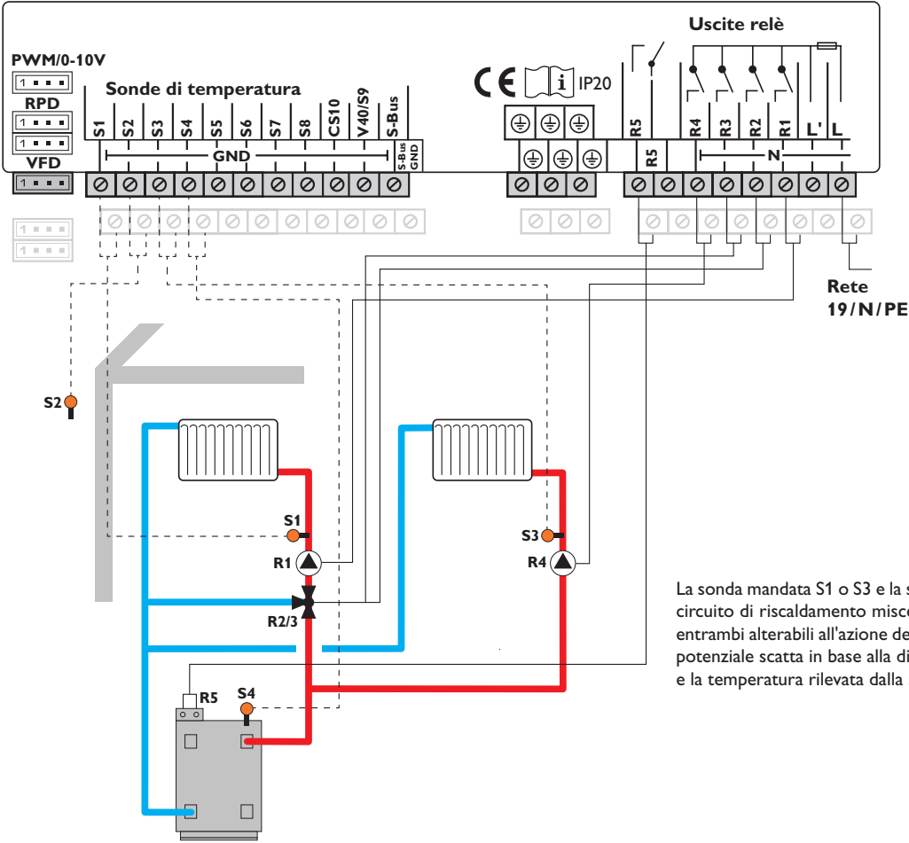
Schema 7: un circuito di riscaldamento miscelato e un circuito di riscaldamento diretto con riscaldamento integrativo (richiesta)
