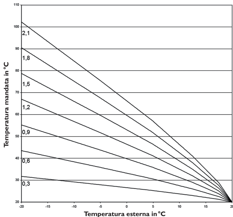
Curve caratteristiche
