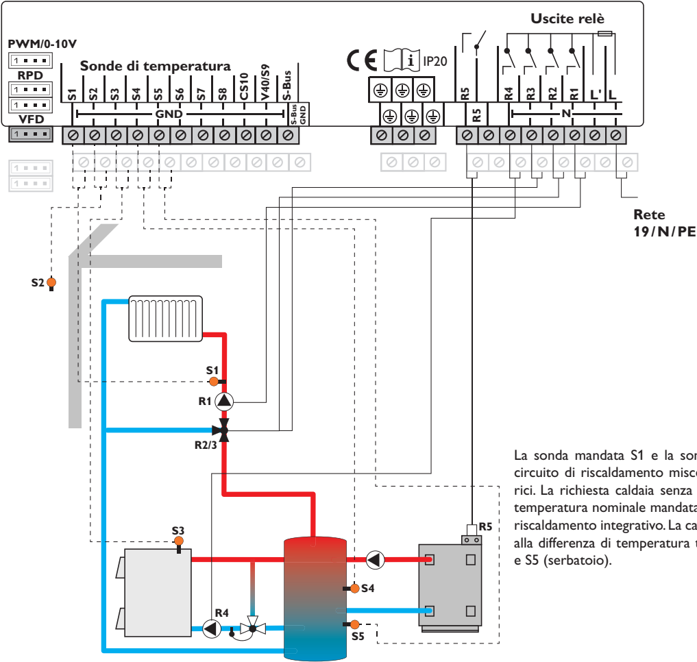
Schema 9: un circuito di riscaldamento miscelato con caldaia a combustione solido e riscaldamento integrativo (richiesta)
