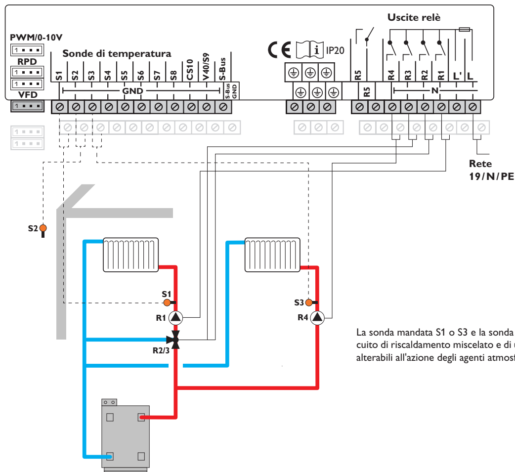
Schema 6: un circuito di riscaldamento miscelato e un circuito di riscaldamento diretto
