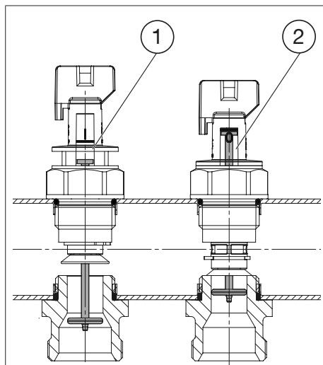
Fig. 5: Setarea indicatorului de debit
