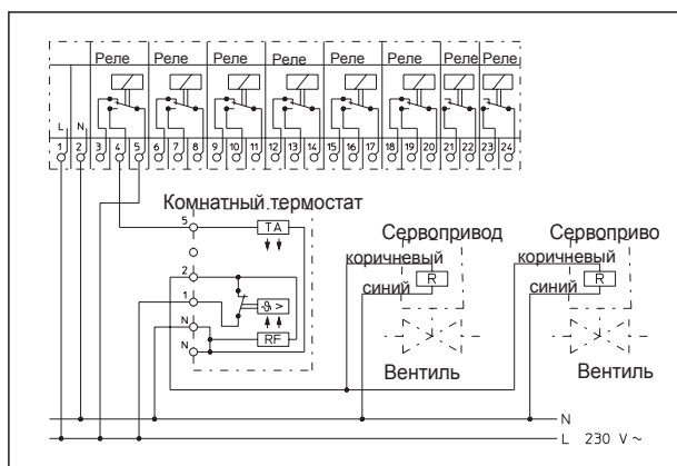
Схема переключения
