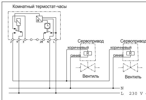
Схема переключения
