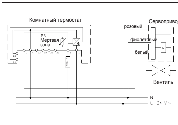
Схема переключения
