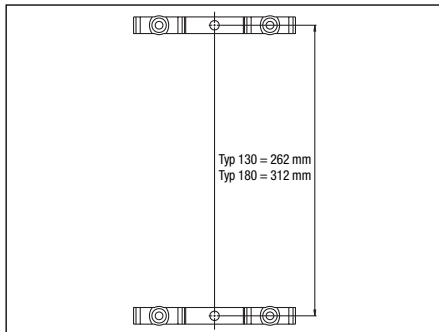
2. Zur Wandbefestigung zwei 8 mm Bohrungen in einem Abstand von 262 mm („Regusol-130“) bzw. 312 mm („Regusol-180“) anbringen und die beiliegenden Dübel in die Bohrlöcher einsetzen. Dabei die hintere Isolierschale (4) als Bohrschablone einsetzen.
