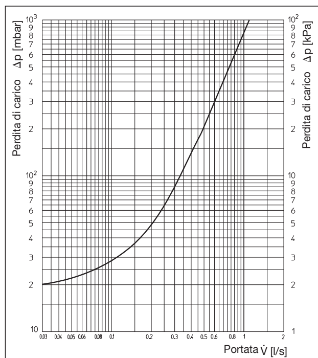
Diagramma delle portate „Regumat RTA-180“ DN 25
