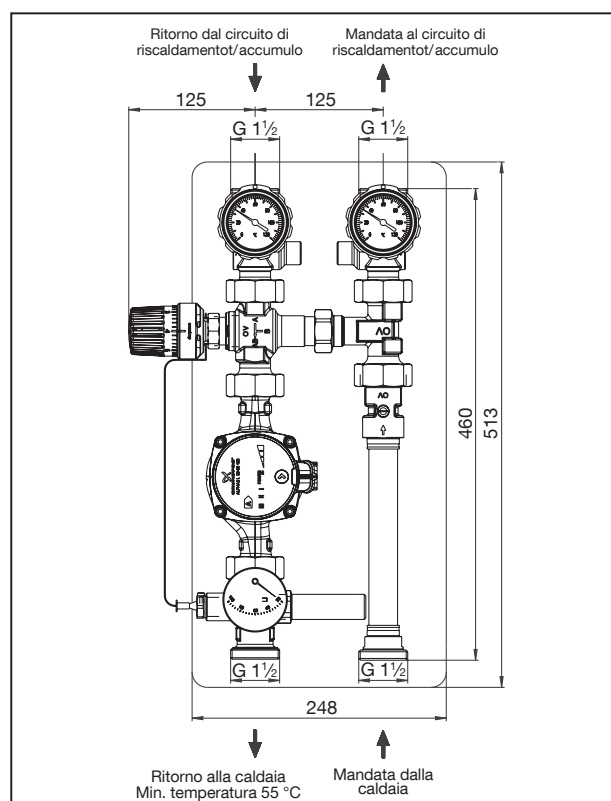
Dimensioni „Regumat RTA-180“ DN 25 con coibentazione standard
