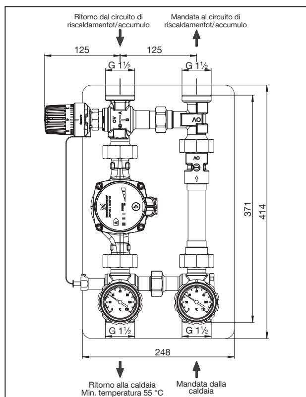
Dimensioni „Regumat RTA-180“ DN 25 con coibentazione universale con struttura modulare
