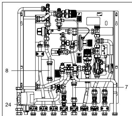
Fig. 6.4 Montaggio contatore acqua fredda e contocalorie
