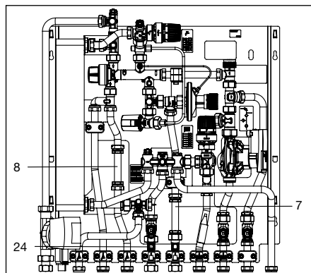
Fig. 6.4 Montage du compteur d'eau froide et du compteur de calories
