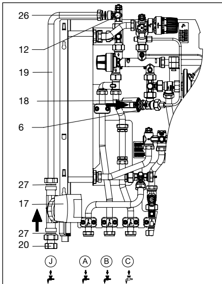
Abb. 6.1 Montage
