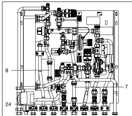
Abb. 6.5 Einbau Kaltwasser- und Wärmezähler
