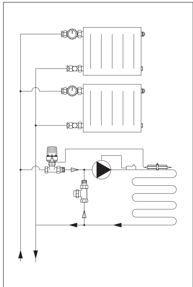
System-Darstellung
