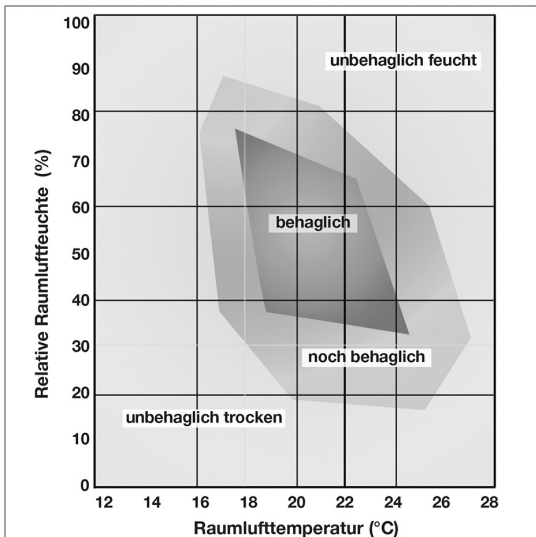
Abb. 59: „Behaglichkeitsdiagramm“
