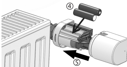
Abb. 56: Batteriewechsel Stellantrieb
