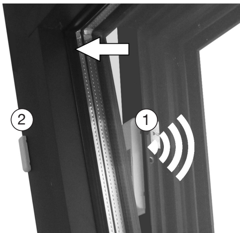
Abb. 23: Auslösung Fensterkontakt
