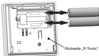
Abb. 53: Batteriewechsel „R-Tronic“
