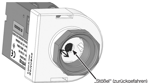
Abb. 11: Montageposition des Aktor-Stößels
