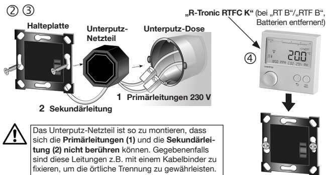
Abb. 7: „R-Tronic“ mit Unterputz-Netzteil 230V
