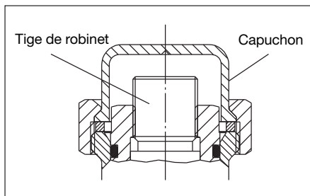
Fig. 7.1: Mécanisme de réglage
