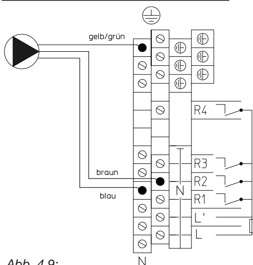
Abb. 4.9: \overline{N} Verdrahtung Zirkulationspumpe mit Regler
