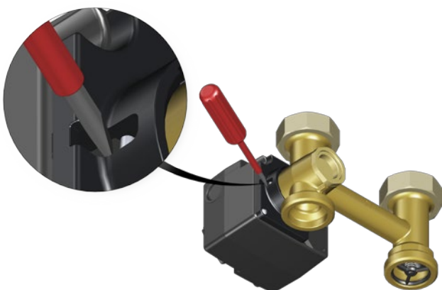
Abb. 30: Stellmotor vom Mischhahn abziehen
