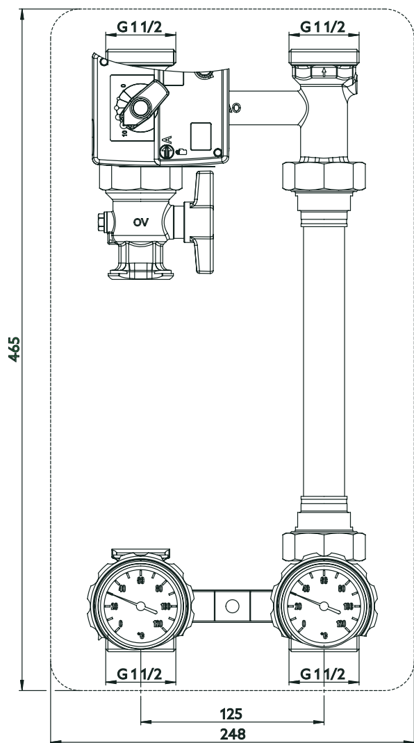
Abb. 20: Vorderansicht
