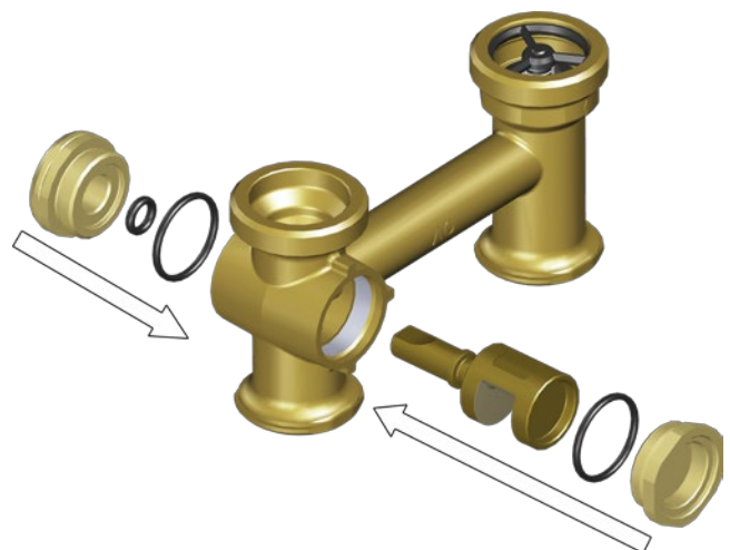
Abb. 36: Mischhahn montieren
