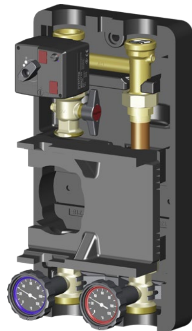
Abb. 24: Armaturengruppe eingehängt (Darstellung ohne Pumpe)
