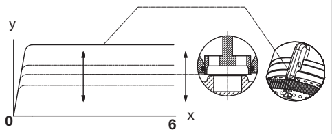
Abb. 4: Pression différentielle p1 – p3 (bar)
