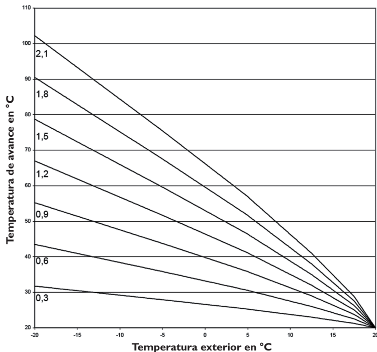
Curvas características de calefacción
