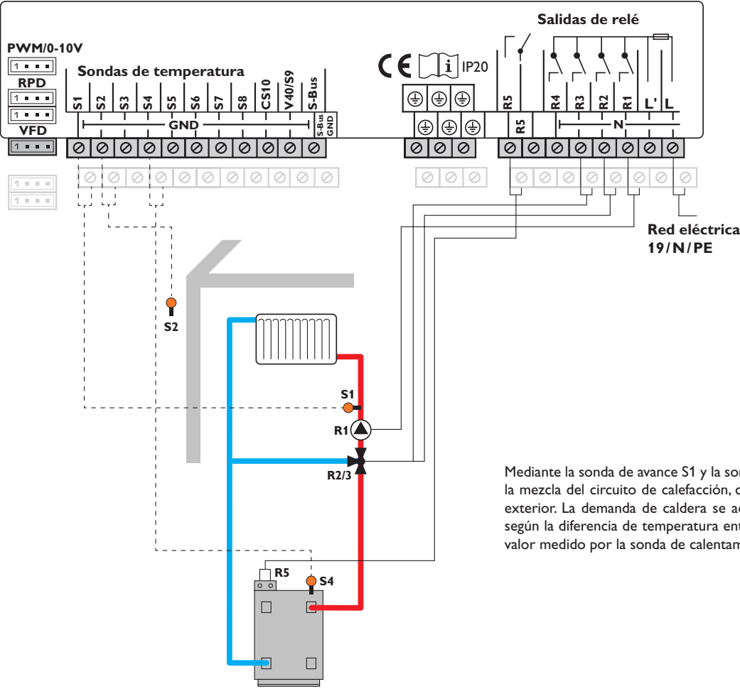
Esquema 2: un circuito de calefacción con mezcla y calentamiento auxiliar (demanda)
