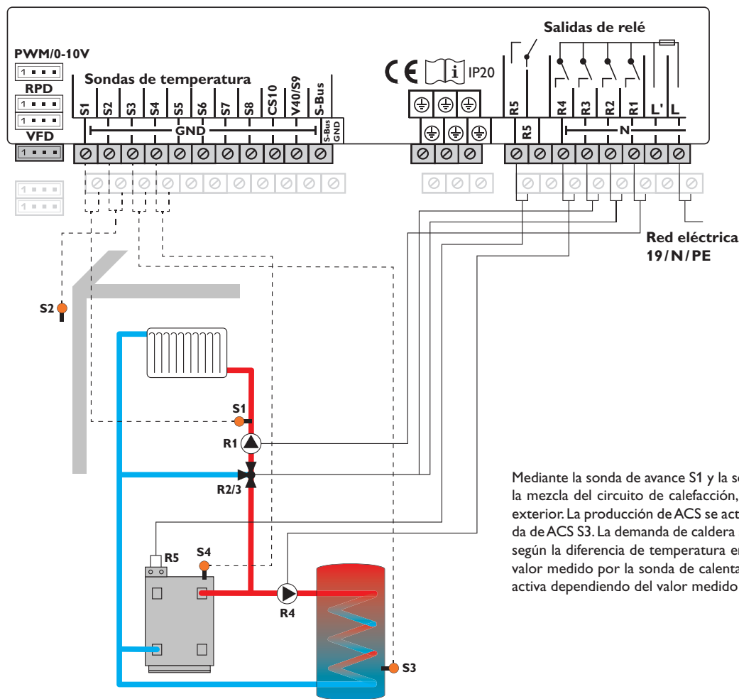
Esquema 5: un circuito de calefacción con mezcla, producción de ACS y calentamiento auxiliar (demanda para circuito de calefacción y ACS)
