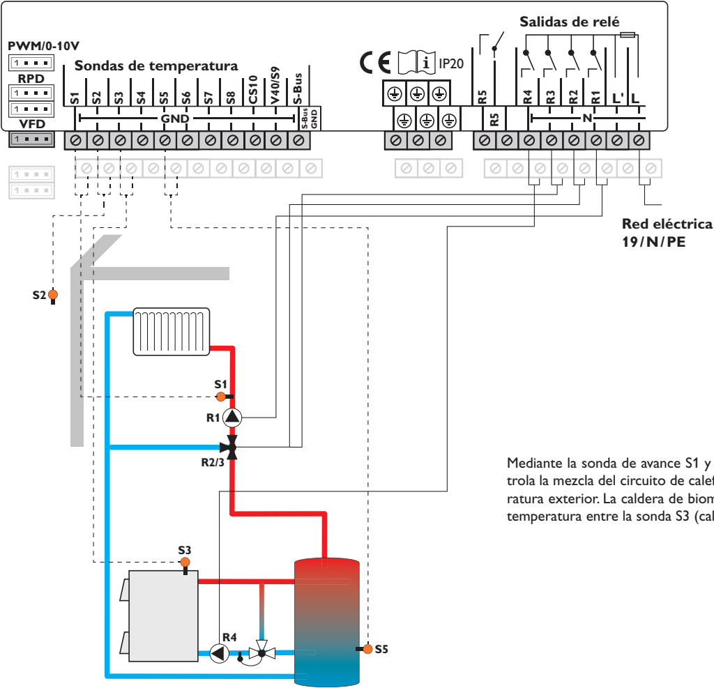
Esquema 8: un circuito de calefacción con mezcla y caldera de biomasa
