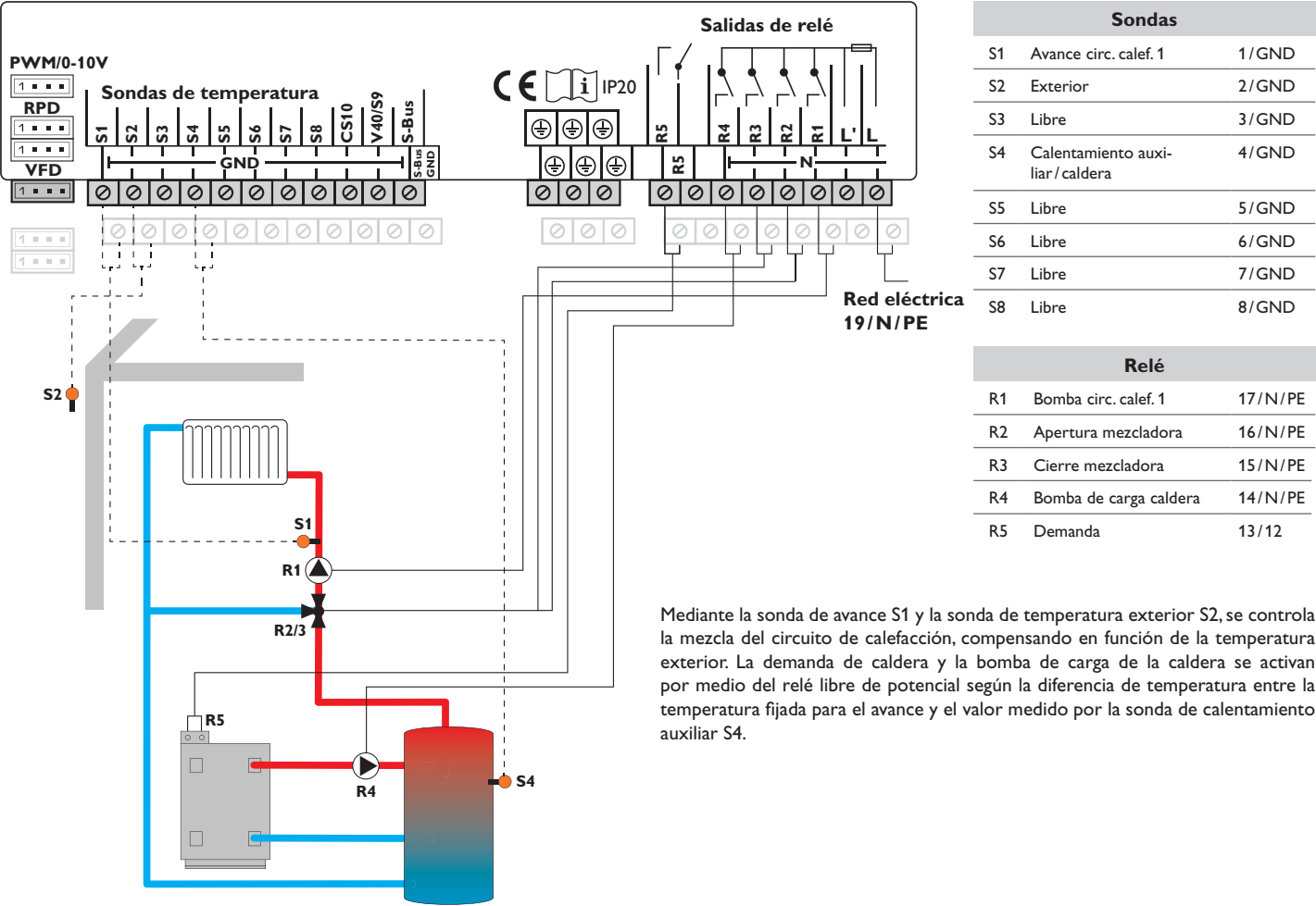
Esquema 3: un circuito de calefacción con mezcla y calentamiento auxiliar (demanda y bomba de carga de la caldera)
