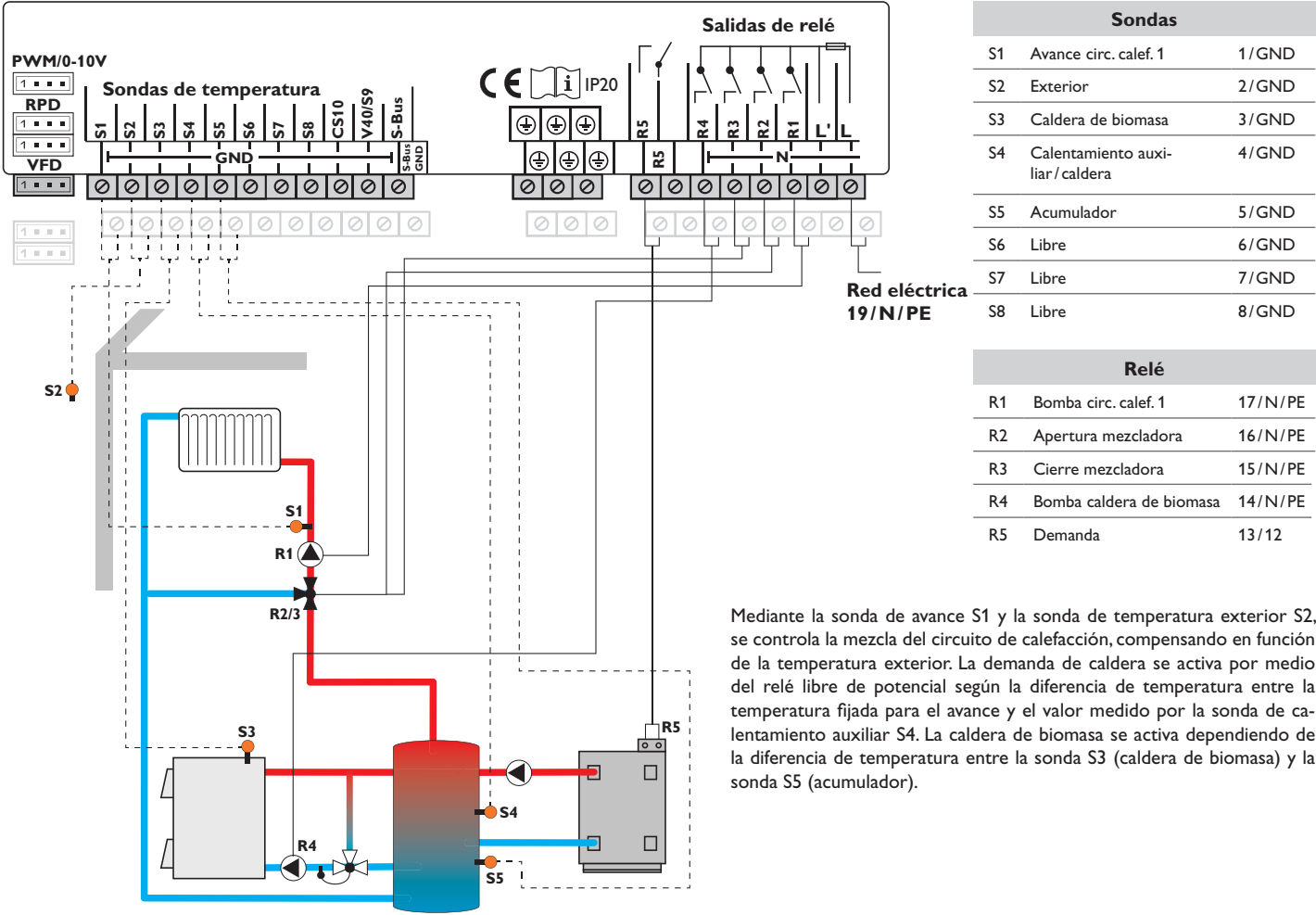
Esquema 9: un circuito de calefacción con mezcla, caldera de biomasa y calentamiento auxiliar (demanda)
