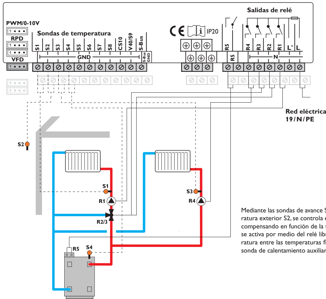
Esquema 7: un circuito de calefacción con mezcla y un circuito de calefacción sin mezcla pero con calentamiento auxiliar (demanda)
