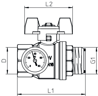
Fig. 5: Encombrements du robinet à tournant sphérique
