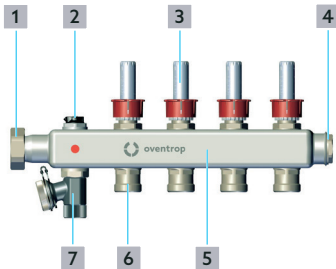
Fig. 1: Aufbau Vorlauf
