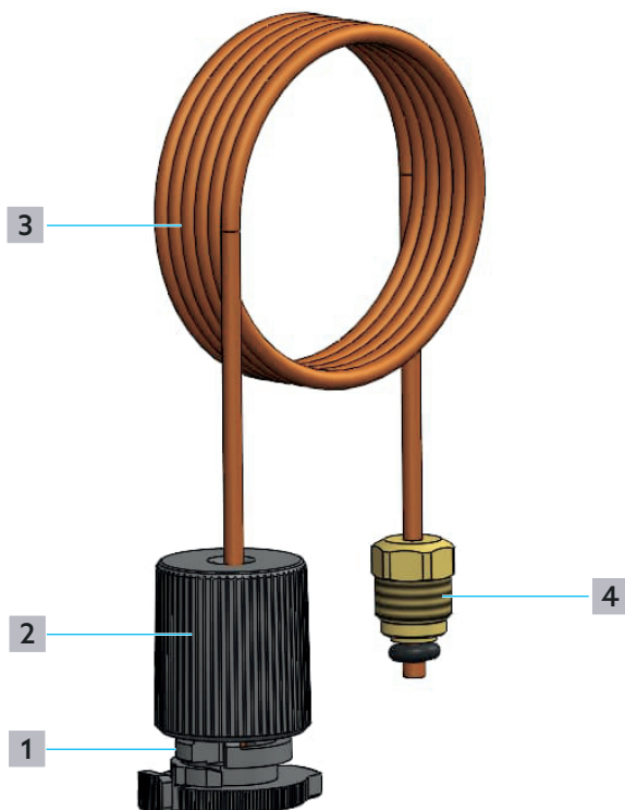
6. Az impulzuscső felépítése
