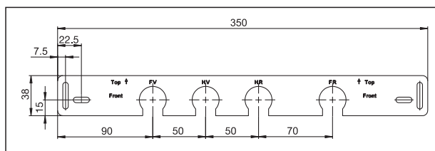
Encombrements du gabarit de montage
