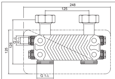
Теплообменник „Regumat“
