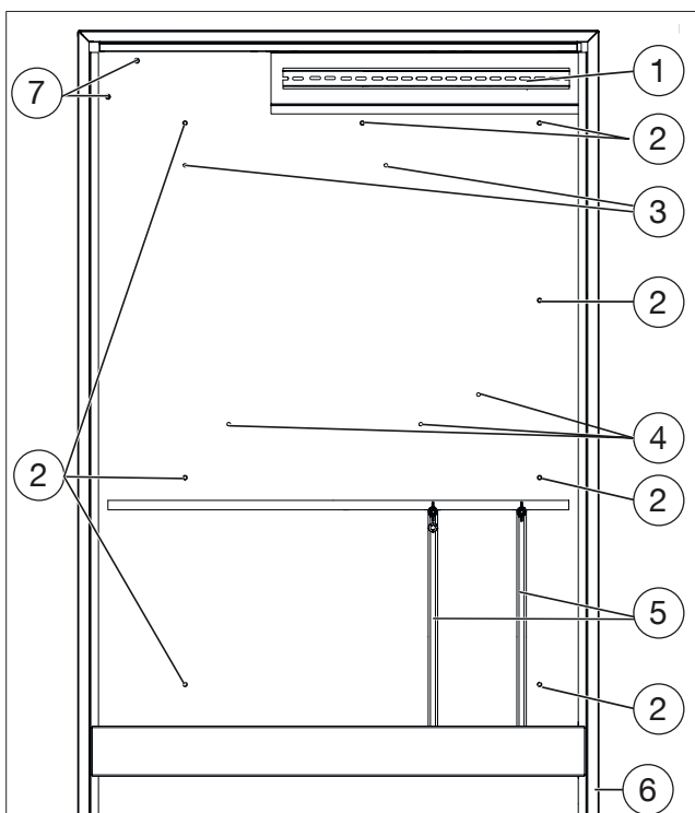
Abb. 2: Aufbau Aufputzschrank 1344698 und 1344699
