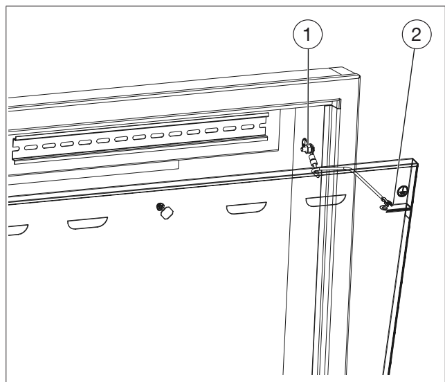
Abb. 8: Erdung der Tür
