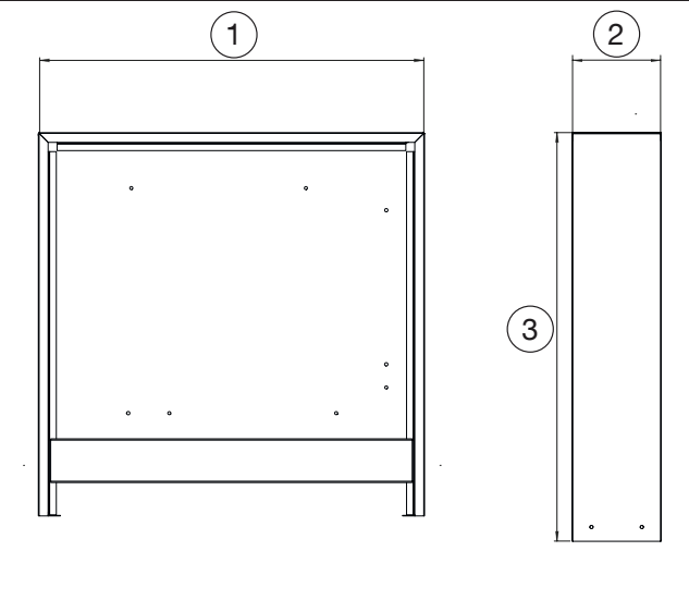
Fig. 4: Dimensions coffret pour pose en applique 1344697
