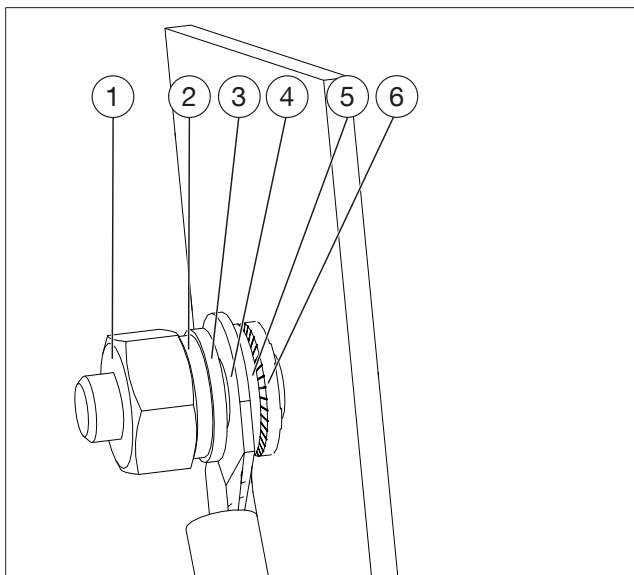
Fig. 9: Construction du point central de mise à la terre
