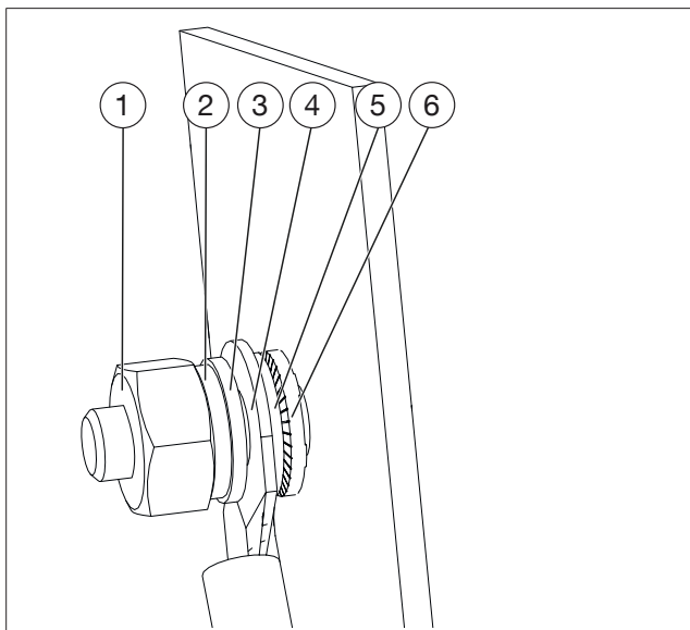
Abb. 9: Aufbau des Zentralen Erdungspunktes
