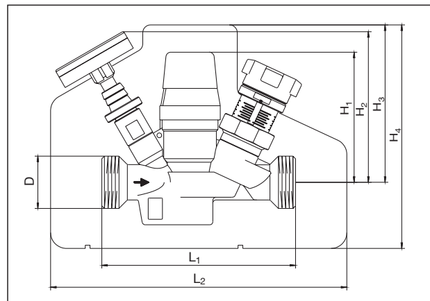
„Aquaström T plus“
