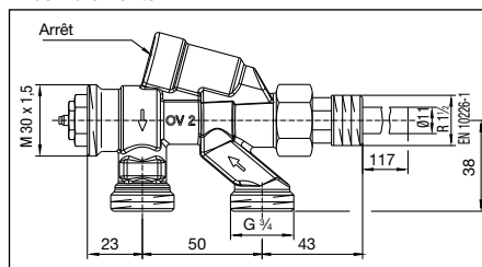
Robinet bitube à plongeur avec lance latérale et arrêt
