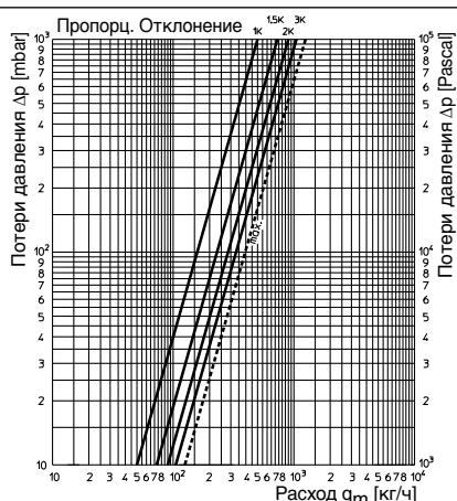
Вентиль Рапира с вертикальной погружной трубкой и функцией отключения
