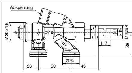
Tauchrohrventil Zweirohr mit seitlicher Lanze und Absperrung
