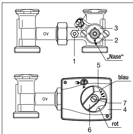
Montage 3-Wege-Mischhahn
