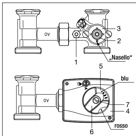
Montaggio del miscelatore a 3 vie
