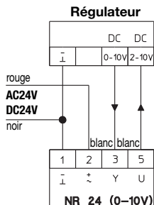
Schéma de branchement
