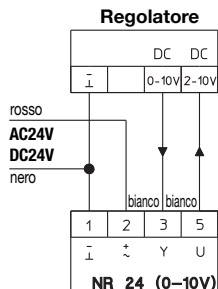
Schema di collegamento elettrico
