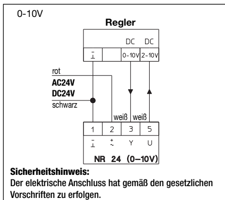
Anschluss-Schema
