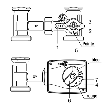
Montage vanne mélangeuse à trois voies
