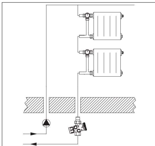
«Unofix QB» (circuit de chauffage vertical)
