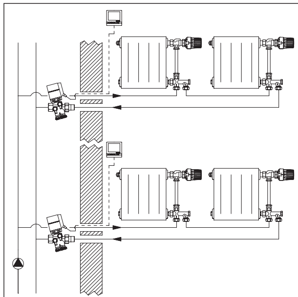
«Unofix QT» (circuits de chauffage horizontaux)
