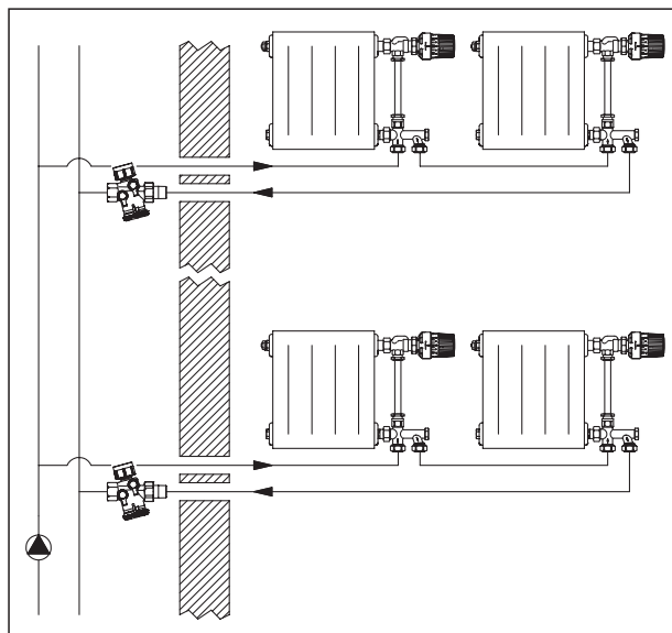
«Unofix QB» (circuits de chauffage horizontaux)
