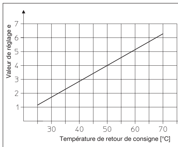
Réglage de la température de retour - valeurs de réglage
