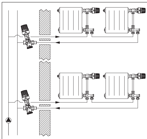
«Unofix QR» (circuits de chauffage horizontaux)
