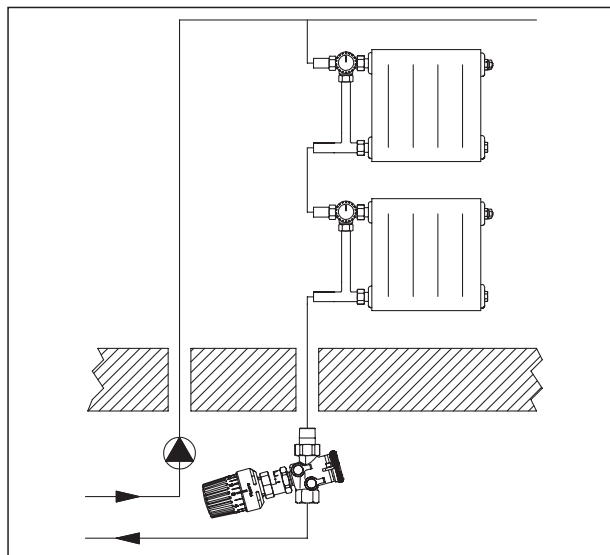
«Unofix QR» (circuit de chauffage vertical)
