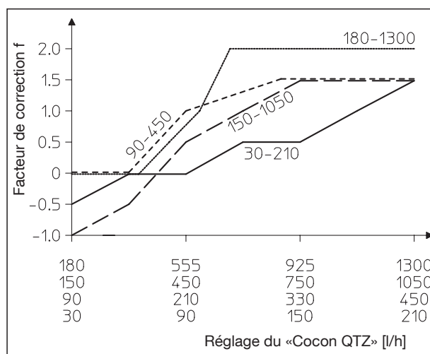
Réglage de la température de retour- facteur de correction f
