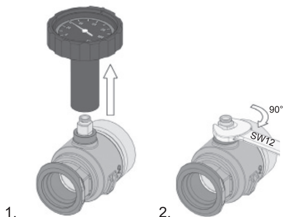
Рис. 21: Закрывание шарового крана
