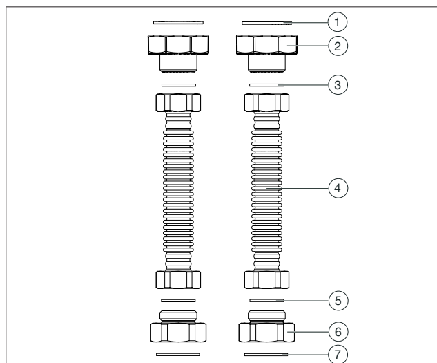
Abb. 29: Aufbau Verbindungsset
