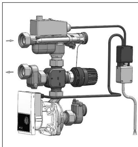
Fig. 1.1 Gruppo di regolazione “Regufloor HN”
