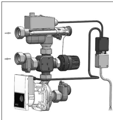
Abb. 1.1 „Regufloor HN“ Regelstation
