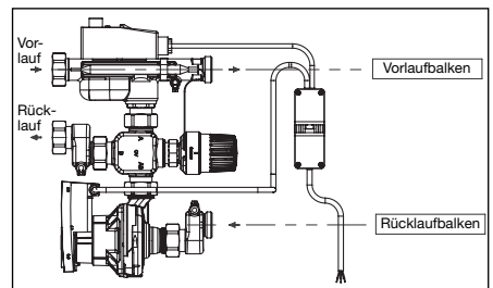
Abb. 6.2 Durchflussrichtung
