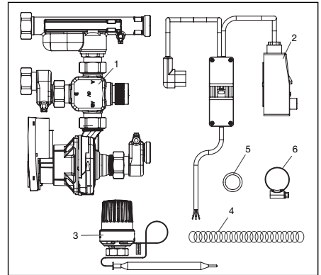
Abb. 6.1 Lieferumfang
