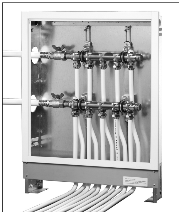
„Multidis SH“ collettore inox
