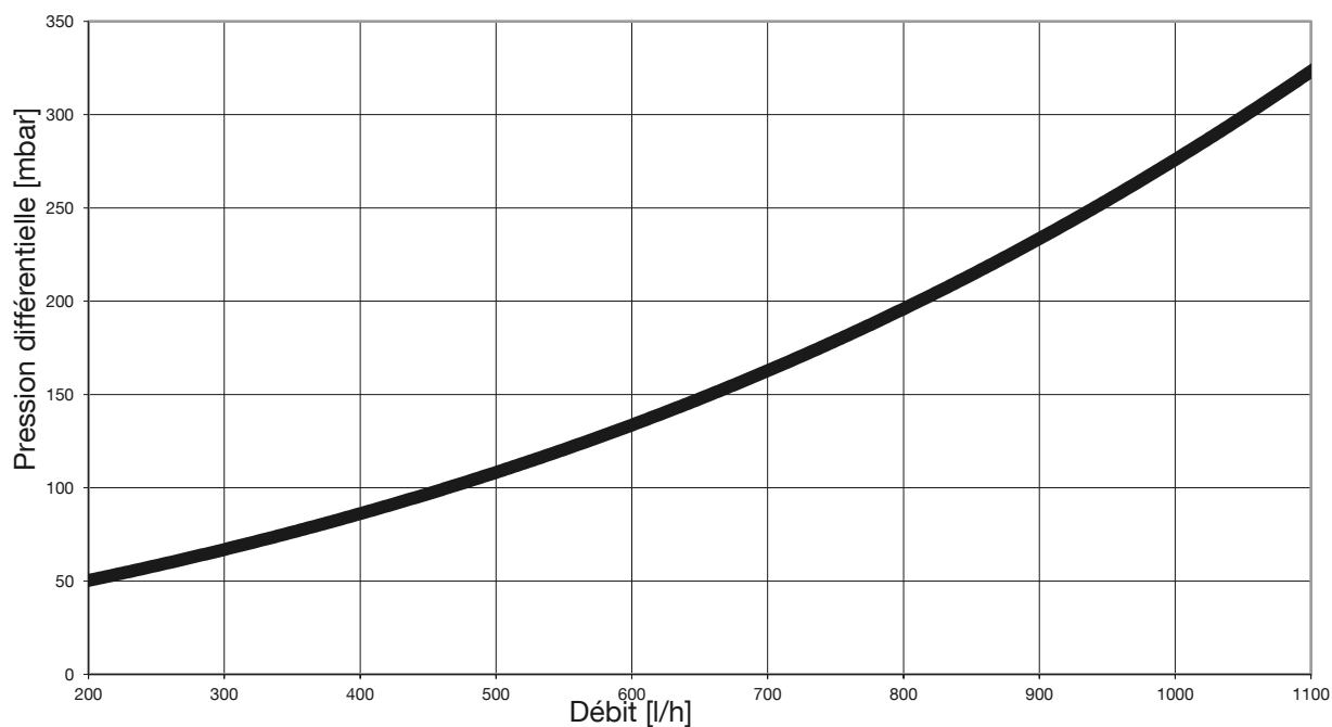
Fig. 5: Perte de charge circuit secondaire Regudis H
