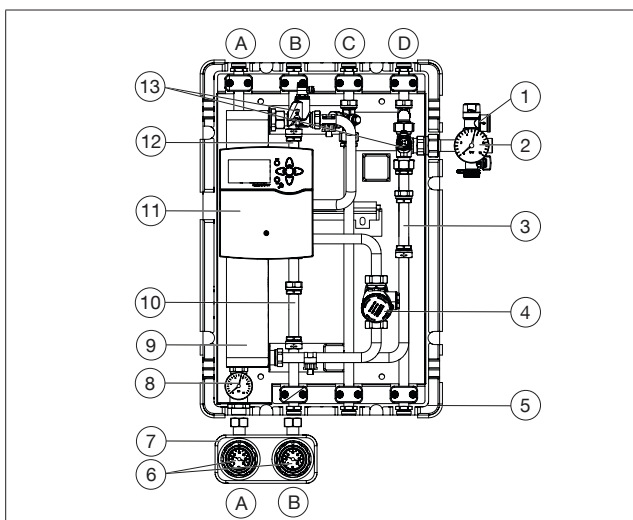
Fig. 2: Configuration Regudis H
