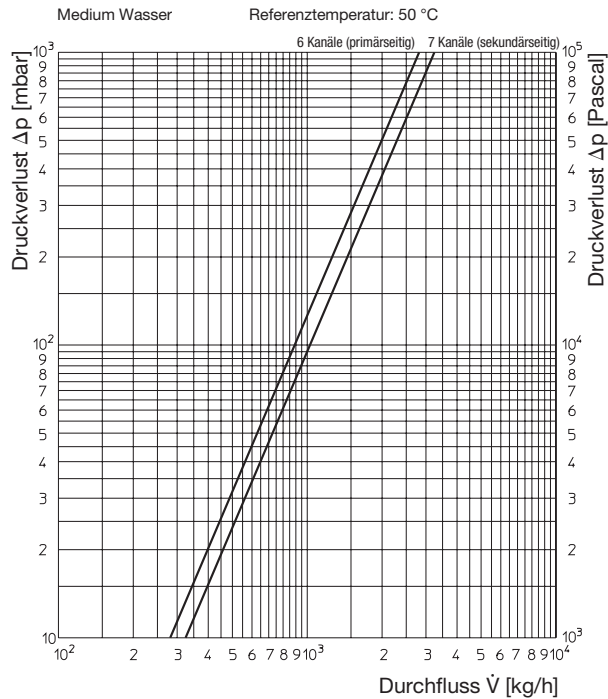
Diagramm Wärmeübertrager
