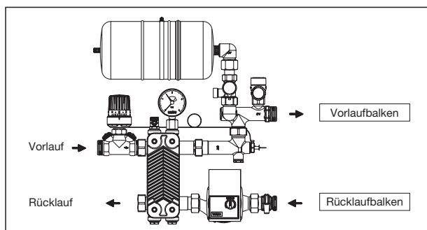
Durchflussrichtung
