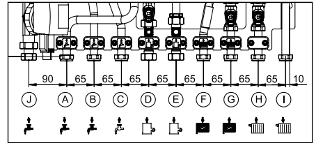
Abb. 4.3 Anschlussmaße
