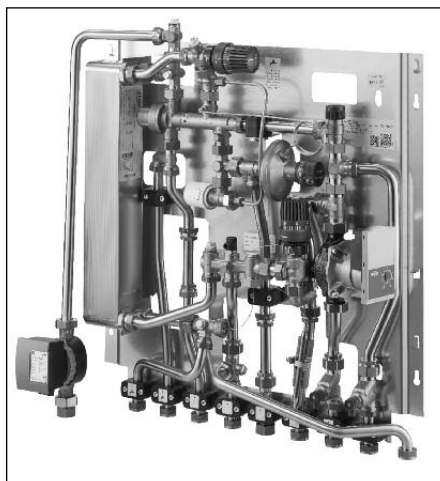
Fig. 1.1 “Regudis W-HTF” Modulo satellite per abitazione con circuito alte temperature e ricircolo
